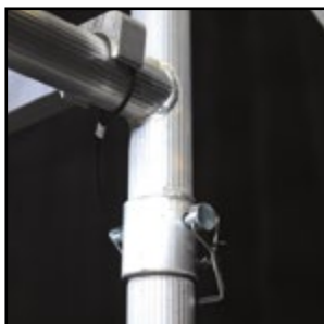
CROCHET DE BARRE. TIGES DE VERROUILLAGE POUR CADRE
